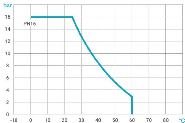
نمودار فشار - دما برای عمر مفید ۲۵ ساله
