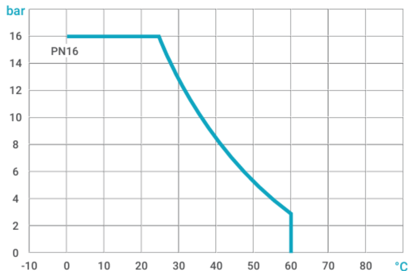
نمودار فشار - دما برای عمر مفید ۲۵ ساله
