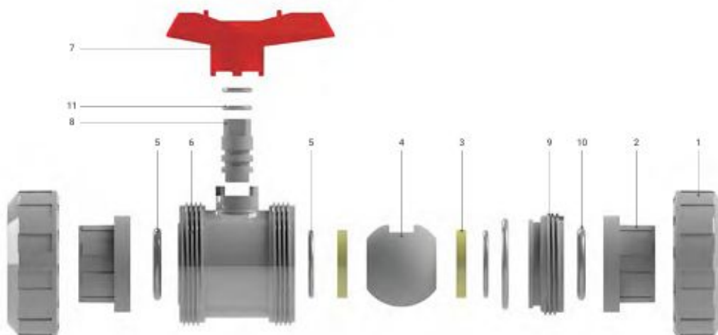
اجزای شیر توپی مهره ماسوره‌ای دوسره‌ای دنده C-PVC
