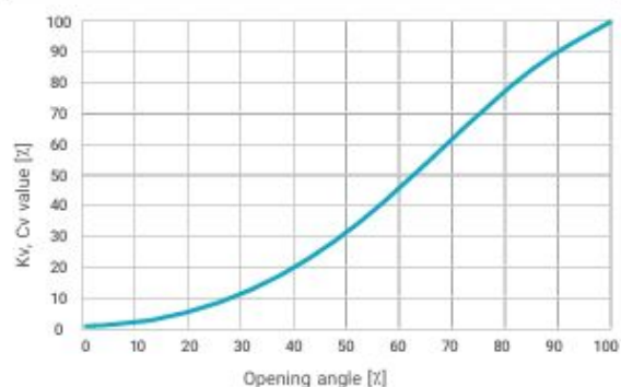
نمودار فاکتور اصلاحی برای ضریب جریان
