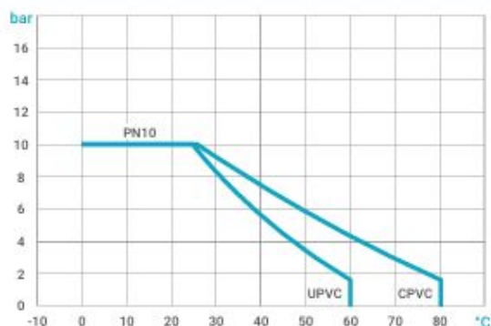
نمودار فشار-دما برای عمر مفید ۲۵ ساله
