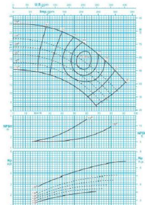
دور موتور ۲۹۰۰ / 2900 rpm
